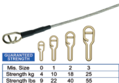
240162 - Stonfo 637 WIRELINK CLIP MIS. 0-1-2-3
