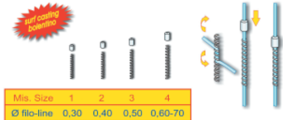
240014 - MOLLA DI STOP - Art. 276
